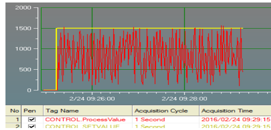
Figure 14. Grafik Nilai KP=100 , KI=10
